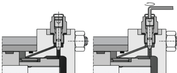
Amortecimento da posição final ajustável com válvula de regulagem do amortecimento
